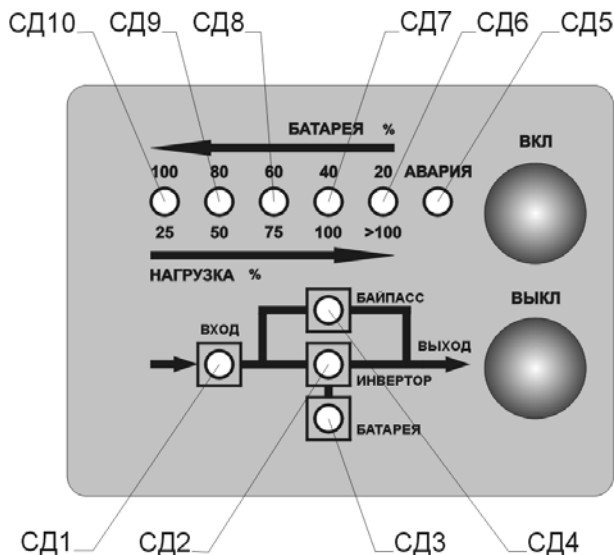
Рис. 1 Передняя панель блока ИБП
