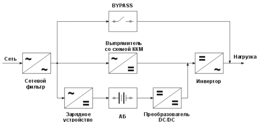
Рис. 2 Структурная схема ИБП
